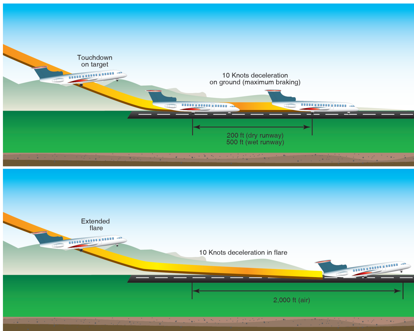
Figure 16-19. Extended flare.
